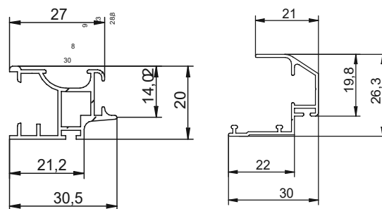
sezione barramaniglia
