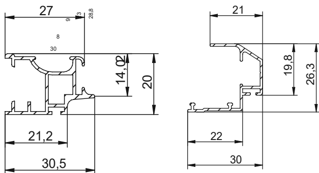
sezione guida
